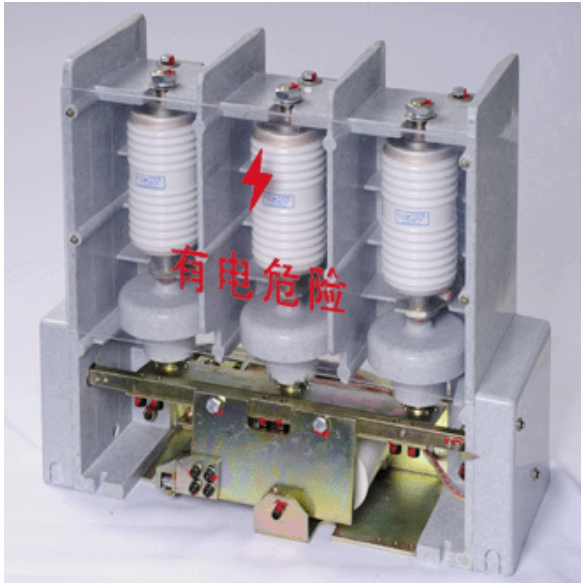
JCZ5-630A/12kV型(电保持)交流真空接触器
